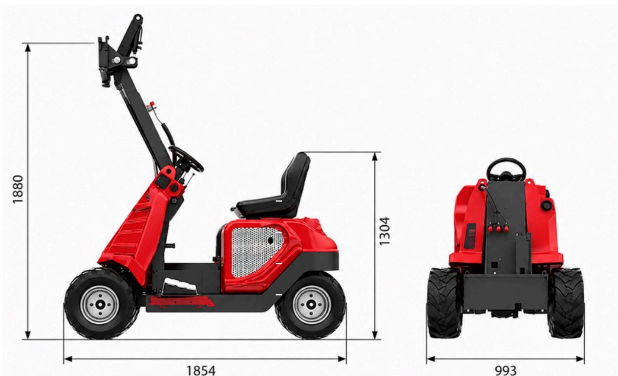
Abbildung zeigt Abmessungen des LG13
