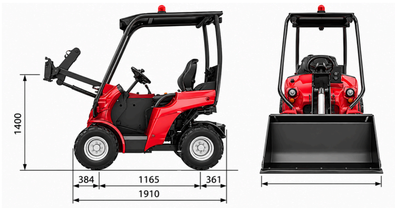
Abbildung zeigt Abmessungen des LG14
