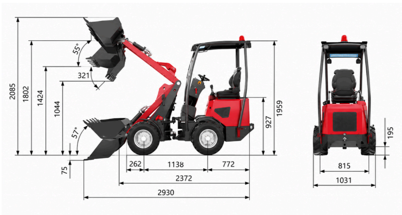
Abbildung zeigt Abmessungen des LG15
