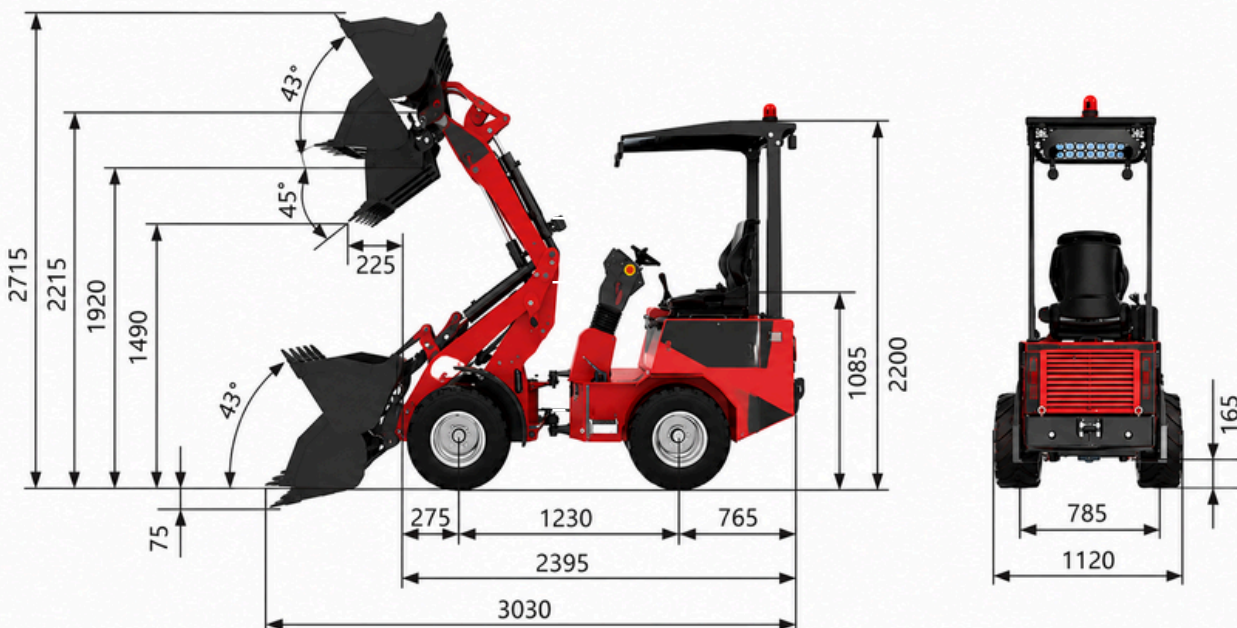
Abbildung zeigt Abmessungen des LG16
