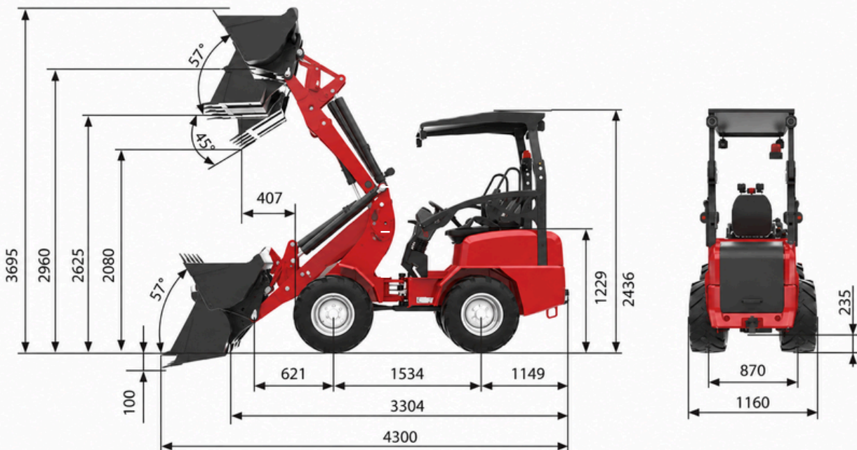
Abbildung zeigt Abmessungen des LG19
