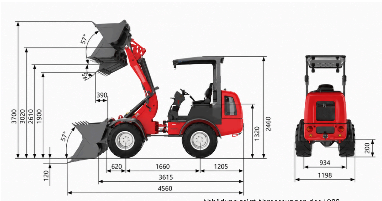
Abbildung zeigt Abmessungen des LG20
