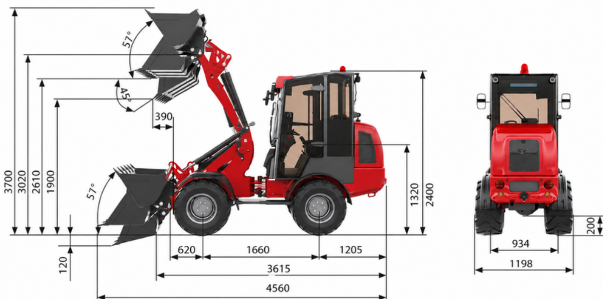
Abbildung zeigt Abmessungen des LG22 *Abhängig von gewählter Sonderausstattung
