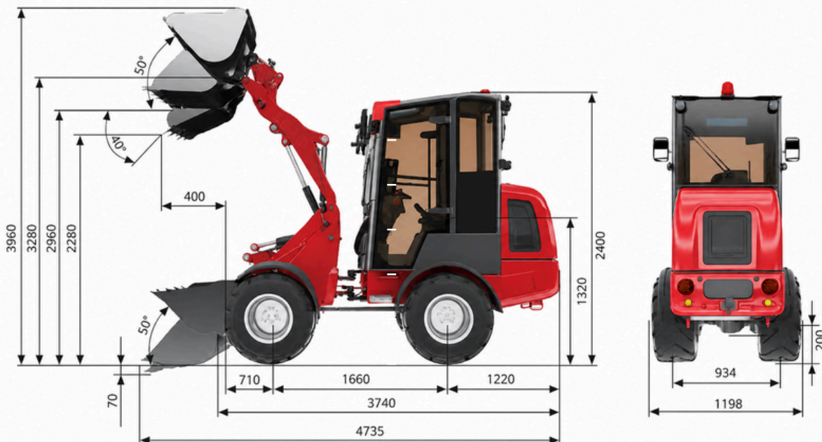
Abbildung zeigt Abmessungen des LG28
