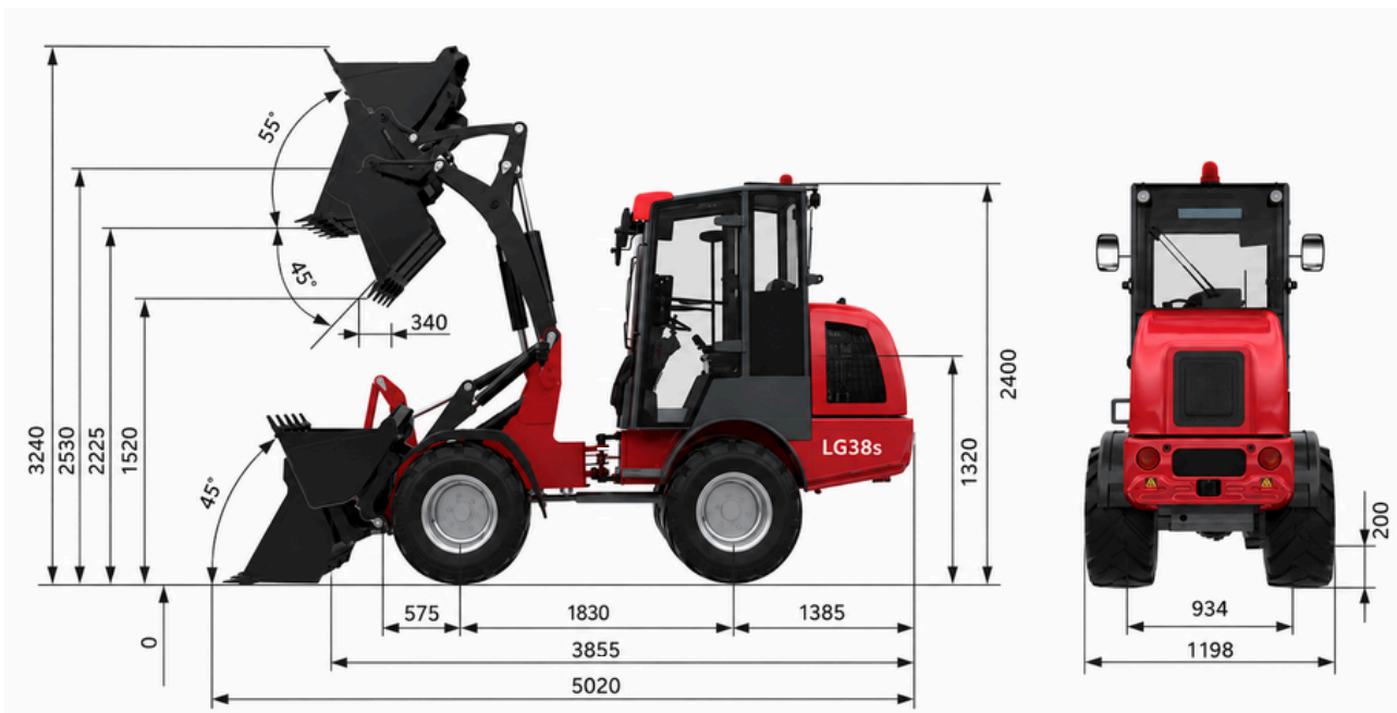
Abbildung zeigt Abmessungen des LG38s
