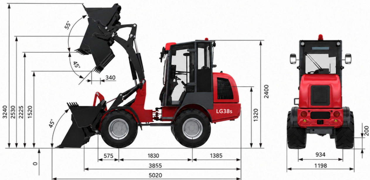
Abbildung zeigt Abmessungen des LG38s *Abhängig von gewählter Sonderausstattung
